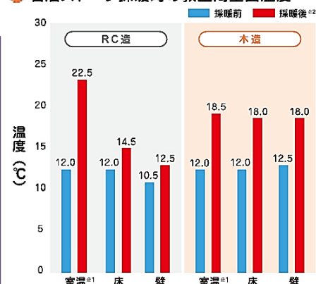
石油ストーブ採暖時の教室周壁面温度
